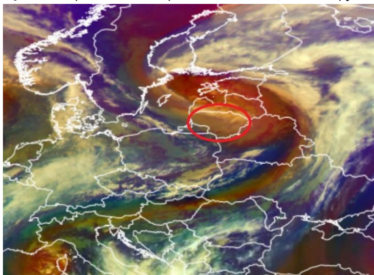
2 pav. Oro masių RGB vaizde šalto oro įsiveržimas (rusva spalva) į Baltijos regioną spalio 9 d. 16 val.
