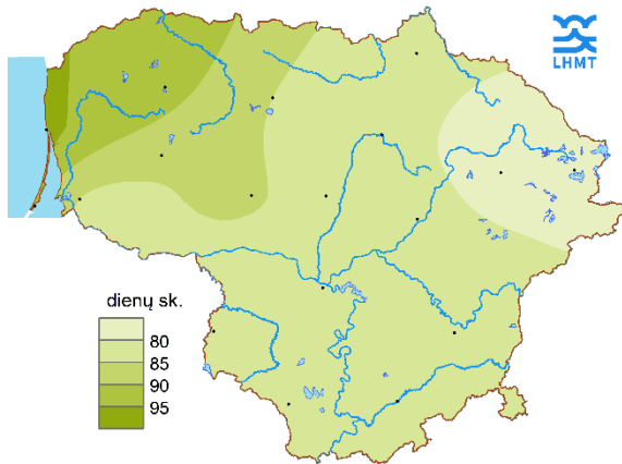
Vidutinė vasaros sezono trukmė, SKN (1961-1990 m.)
