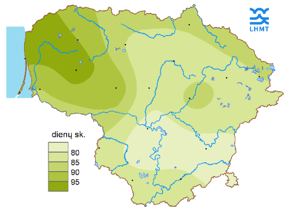
Vidutinė vasaros sezono trukmė, SKN (1991-2020 m.)
