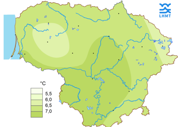
Vidutinē rudenī oro temperatūra, SKN (1991-2020 m.)
