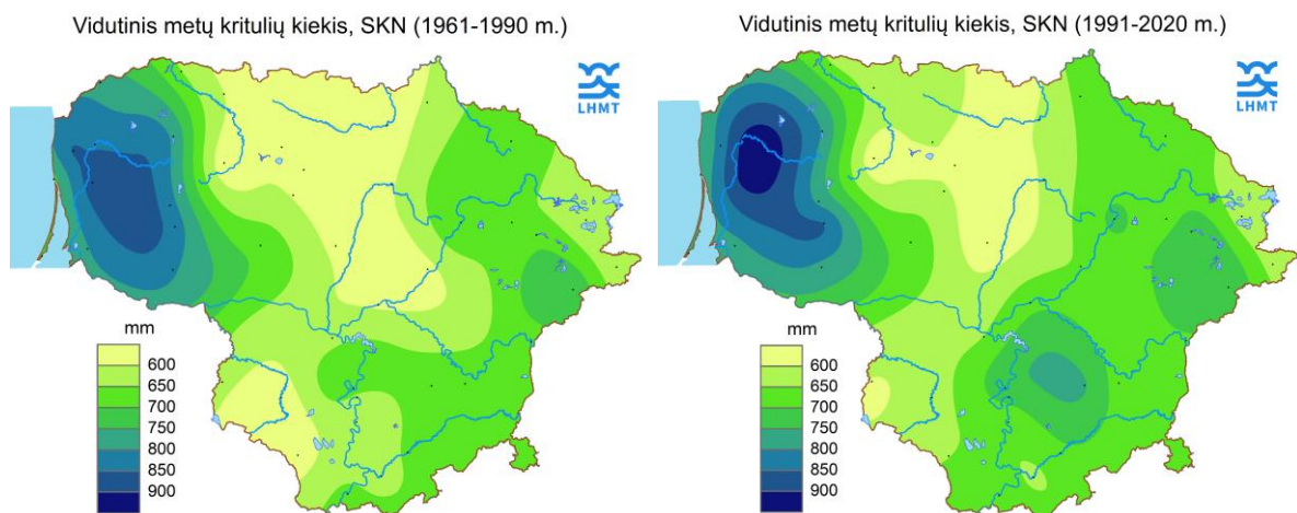
Vidutinio metų kritulių kiekio (mm) Lietuvoje SKN (1961–1990 m.), SKN (1991–2020 m.) ir nuokrypis nuo SKN (1961–1990 m.), %
