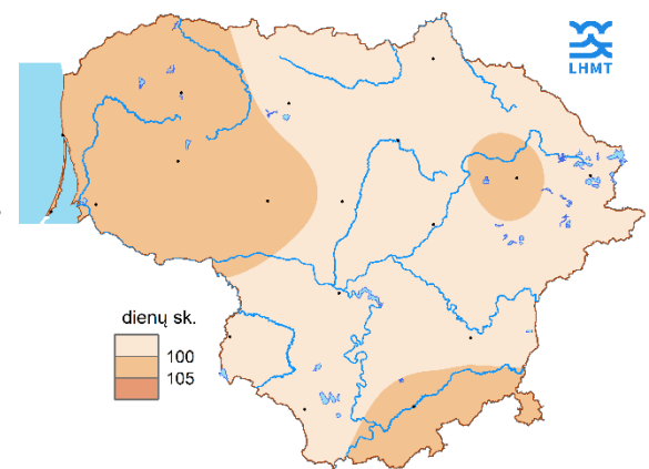
Vidutinė žiemos sezono trukmė, SKN (1991-2020 m.)
