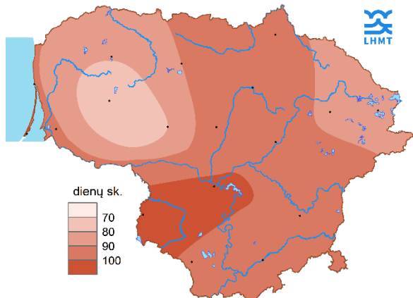
Vidutinė rudens sezono trukmė, SKN (1991-2020 m.)
